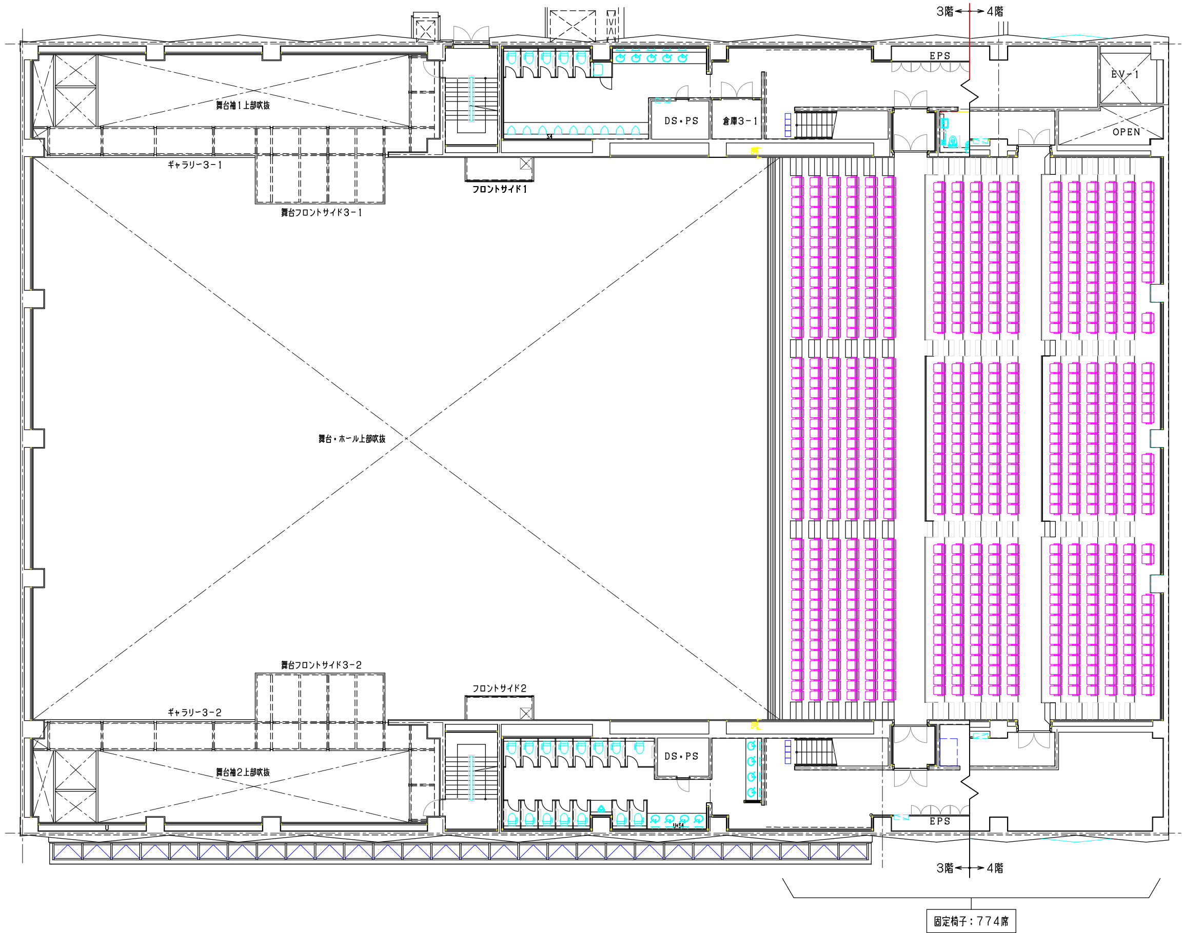
ホール3・4階客席配置図 A1: S=1/100 (A3: S=1/200)
