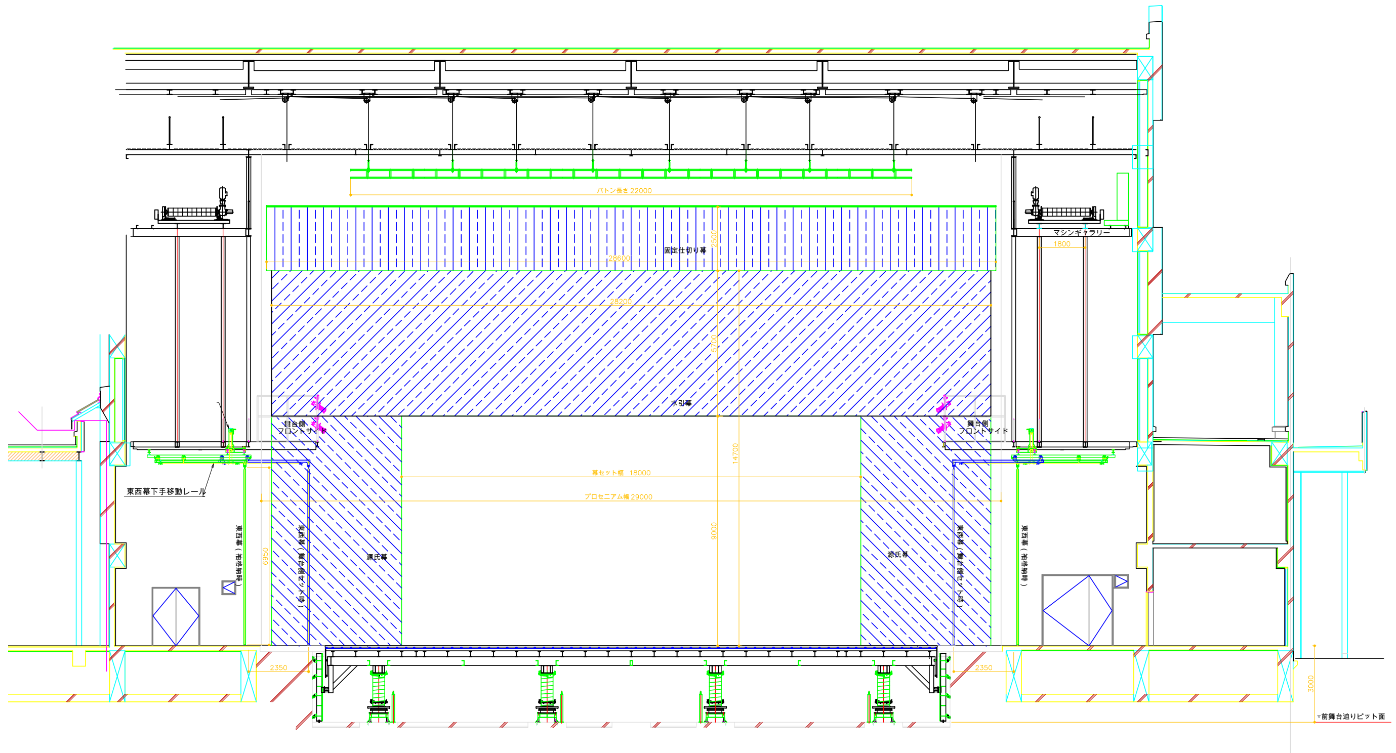
舞台正面図 A1: S=1/75 (A3: S=1/150)
